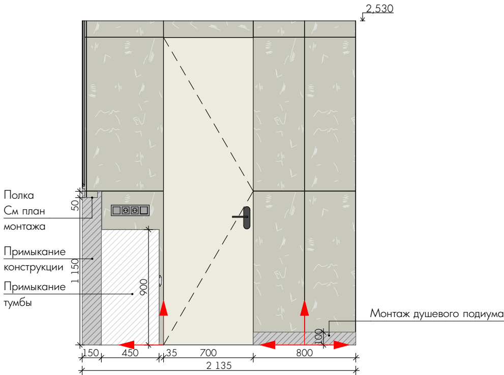
Вид В
