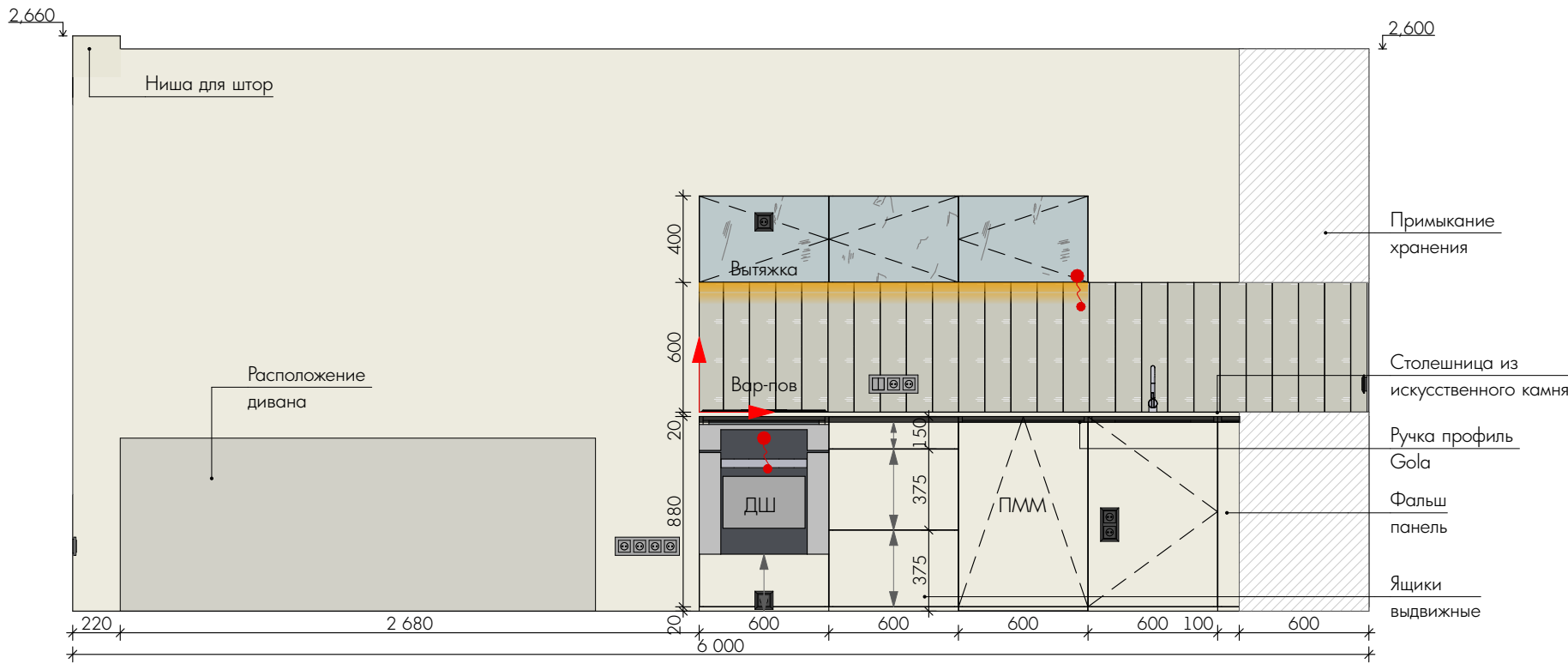
Вид В
