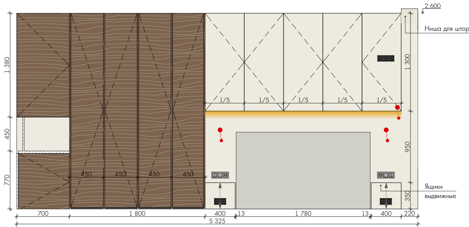
Вид А
