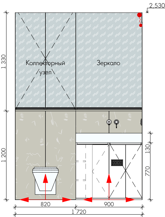
Вид Г
