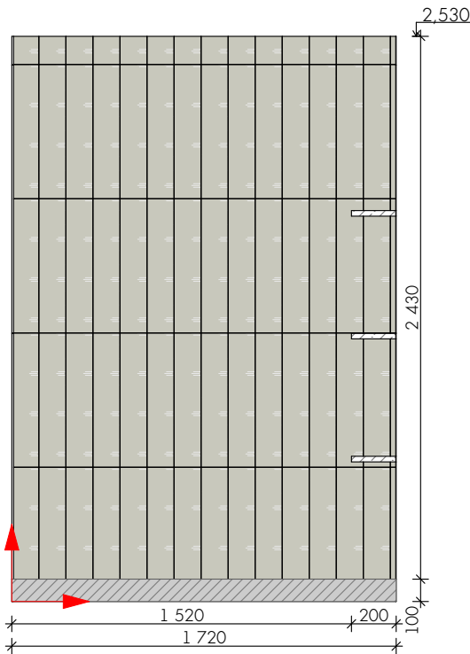
Вид Г
