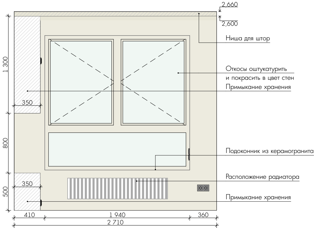
Вид Б
