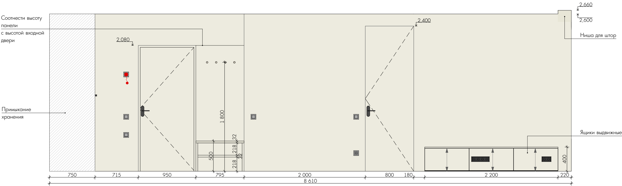
Вид А
