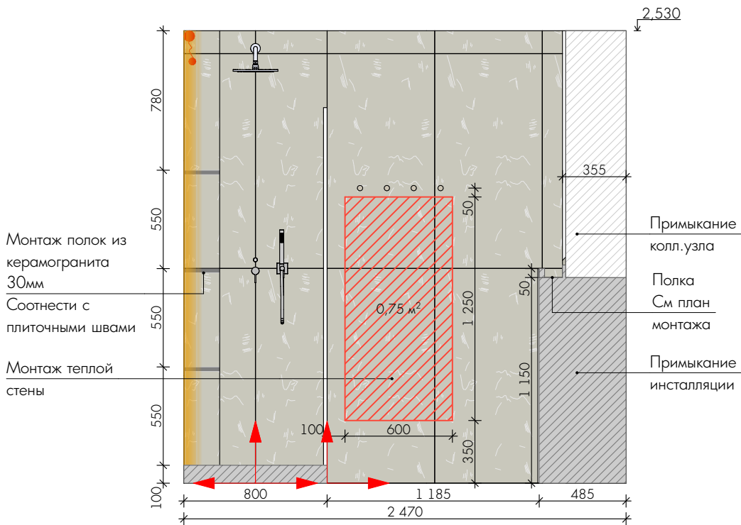
Вид В
